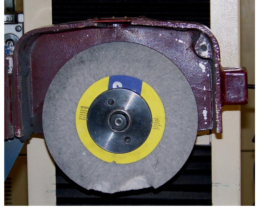
চিত্রঃ ভাঙ্গা গ্রাইন্ডিং হুইল
